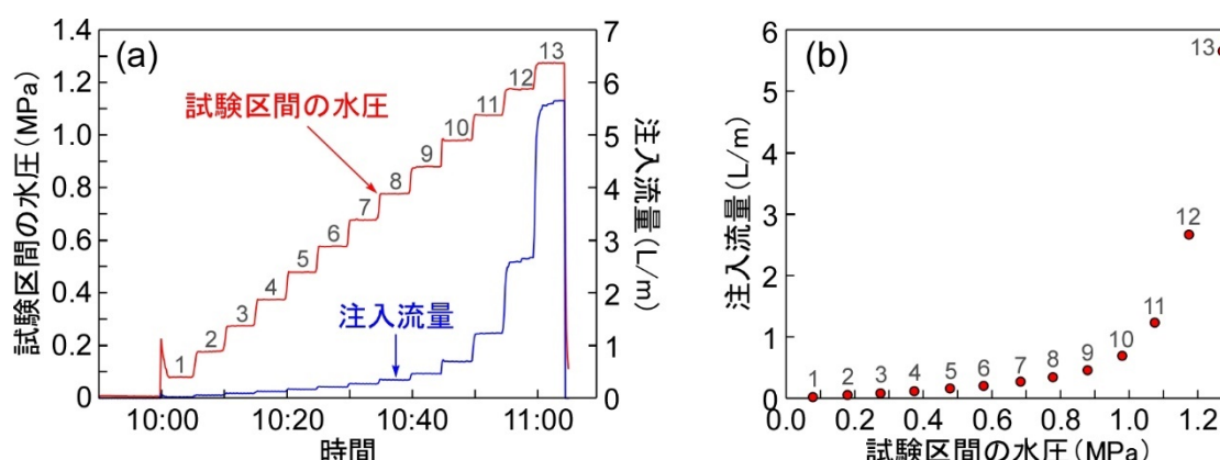
掘削損傷領域の割れ目を対象に実施した既往の注水試験のデータの例
