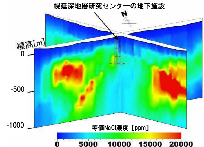
比抵抗分布から推定した等価NaCl濃度の分布 14
