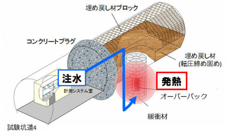
人工バリア性能確認試験の概念図
