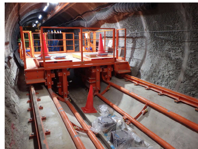
狭隘部の隙間充填装置
