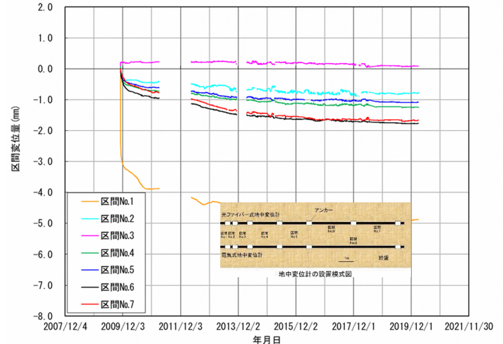
光ファイバー式変位計による計測結果
