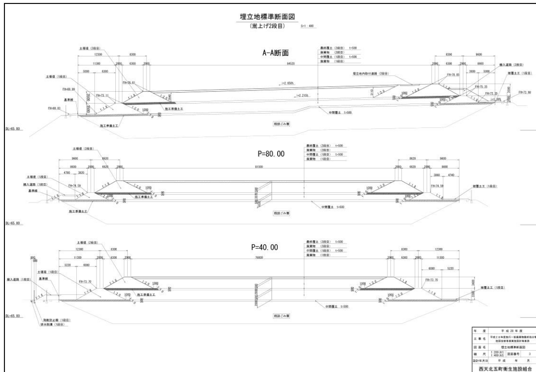
図 2-2 最終処分場断面イメージ
