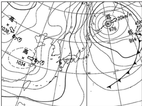
平成 25 年 1 月 8 日の天気図
